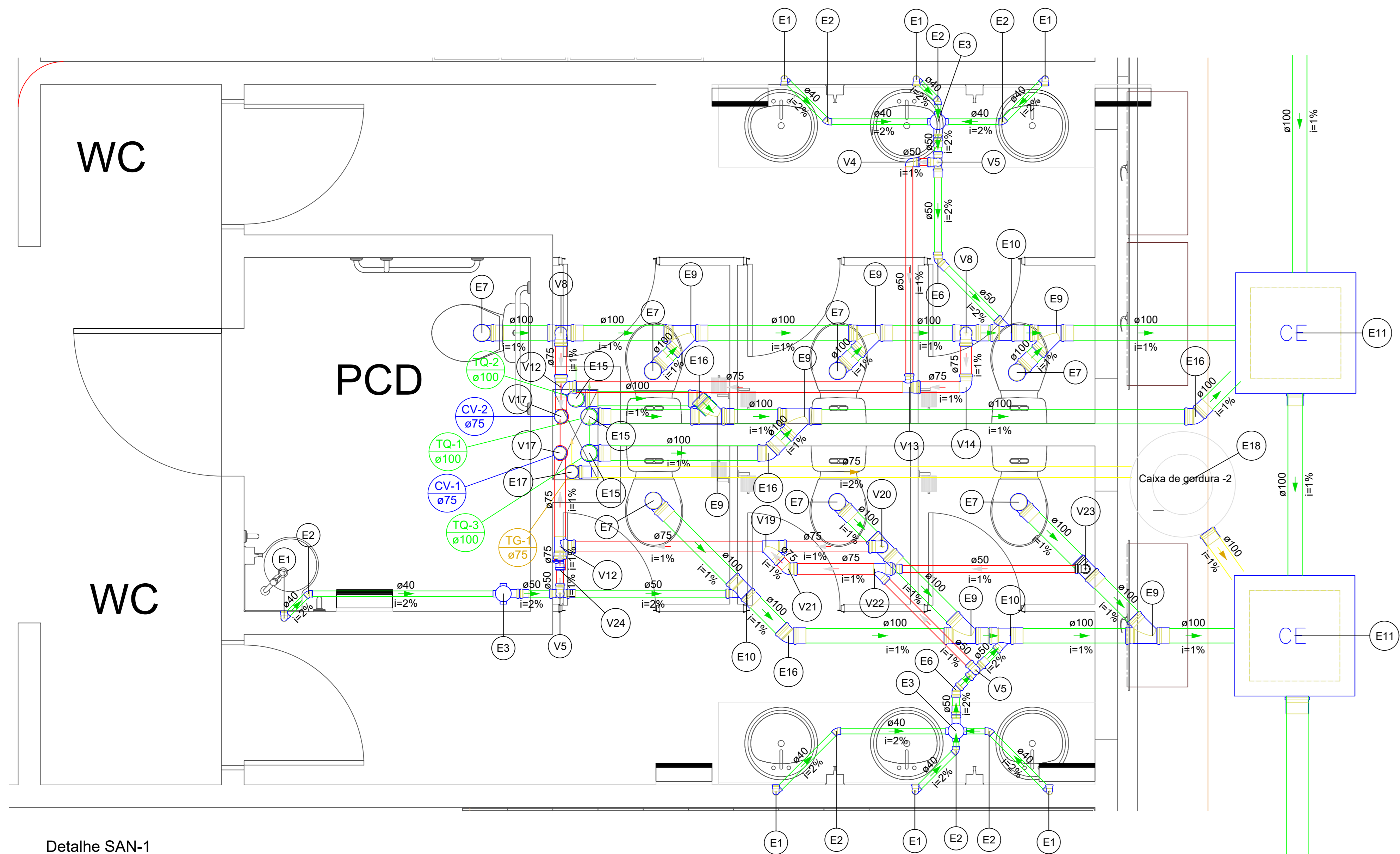
Detalhe SAN-1 Escala 1:25
