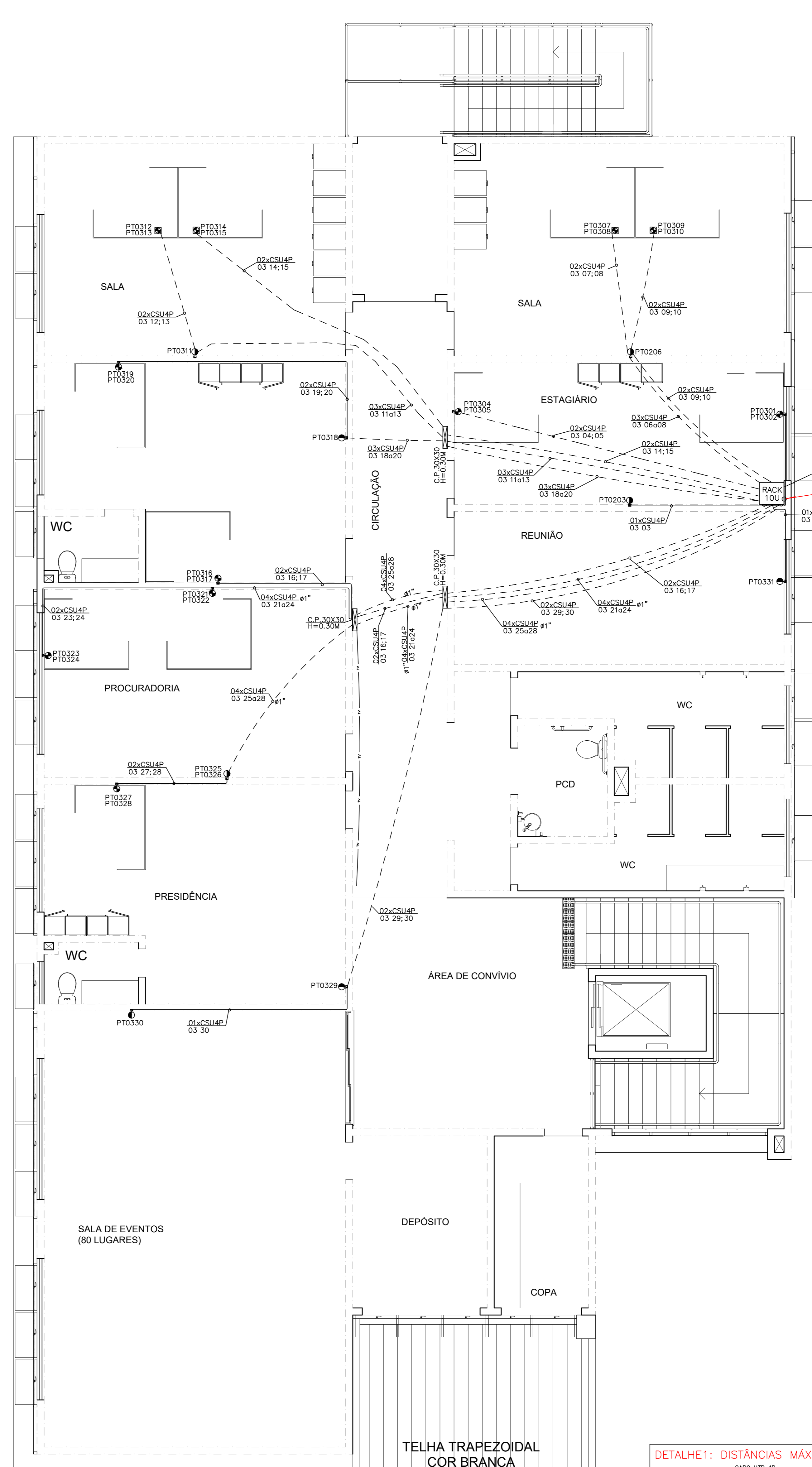
PLANTA BAIXA - 2º PVTO - CABEAMENTO ESTRUTURADO ESC.:1:50
